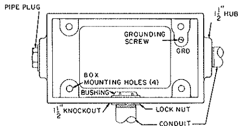
Fig. 4. Conduit box connections
